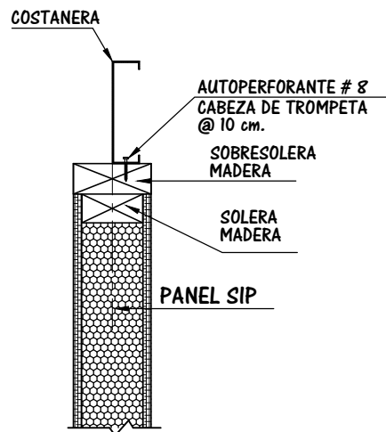
SECCION UNION SUPERIOR PANEL / COSTANERA METALICA
