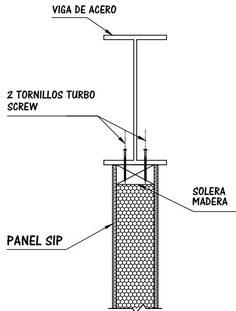
SECCION UNION SUPERIOR PANEL / VIGA IPE
