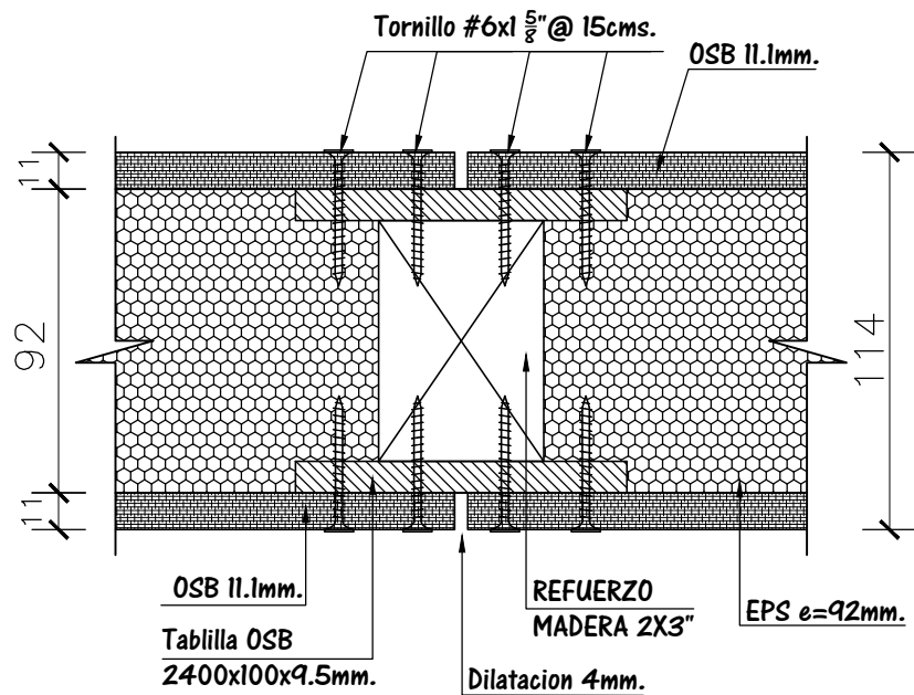
CORTE A-A
