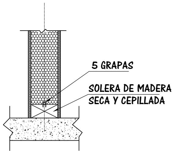
CORTE B-B
