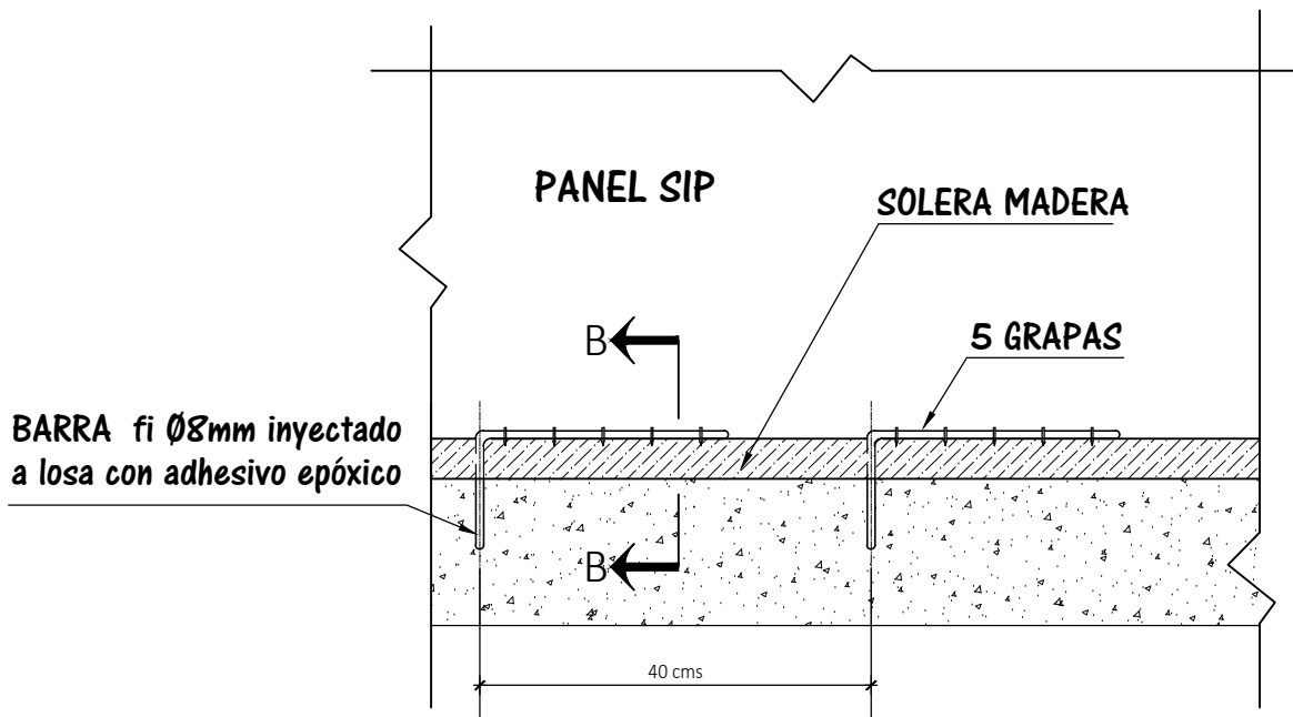
SECCIÓN LONGITUDINAL
